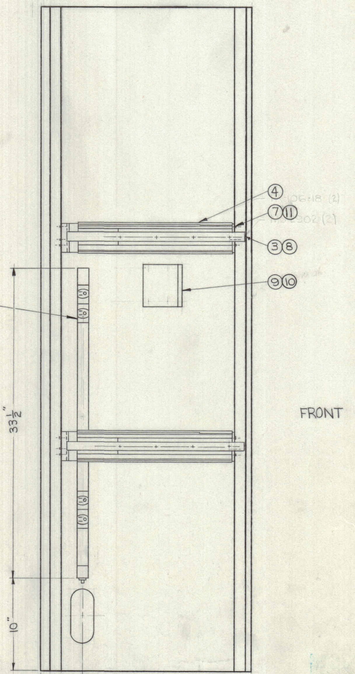
SECTION A-A
